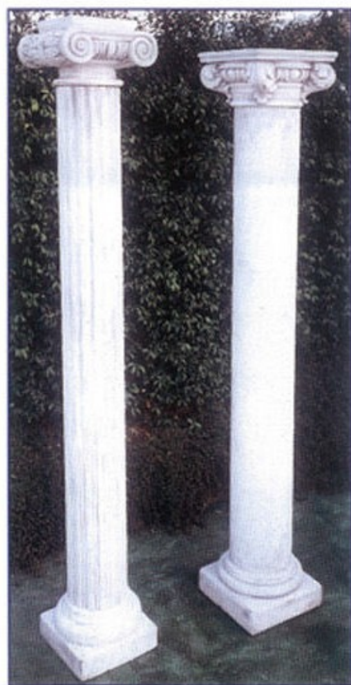
Colonna Corfù ø 27 cm. art. 67 Base cm. 40x40 - Altezza cm. 288 - Peso Kg. 250
